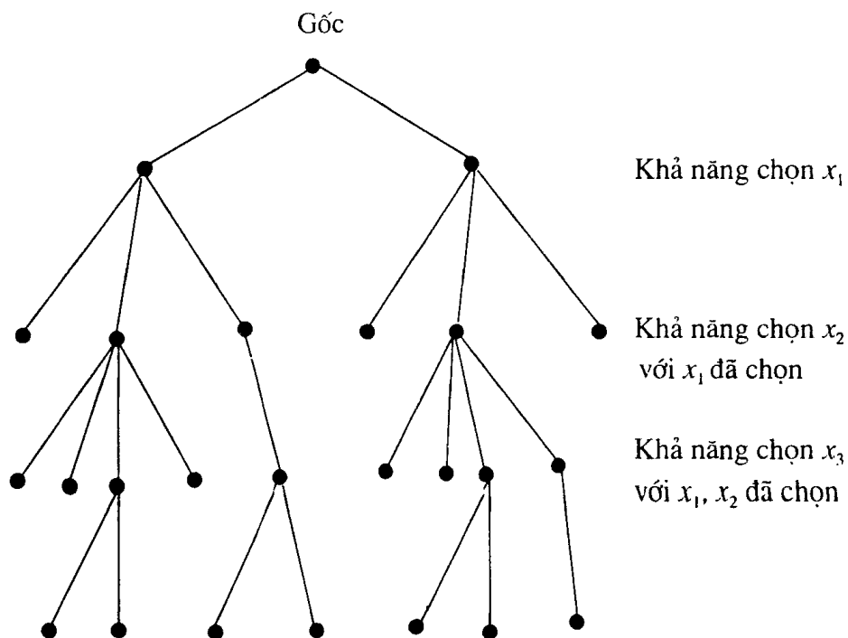
Hình 1. Cây liệt kê lời giải theo thuật toán quay lui
