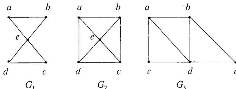
Hình 1. Đồ thị G_1, G_2, G_3
