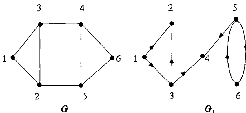
Hình 1. Đồ thị vô hướng G và Đồ thị có hướng G_1
