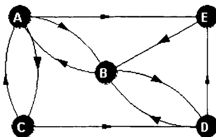
Hình 2. Đồ thị có hướng G
